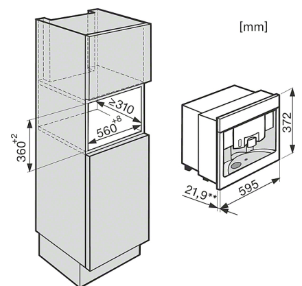
CVA6431ed i högskåp, (skiss) (fotnot)
