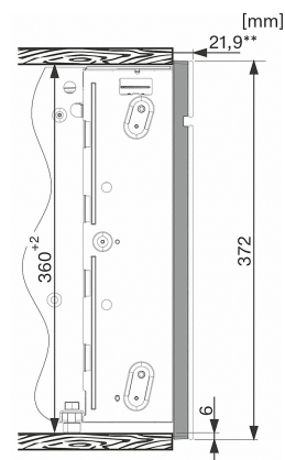
CVA6431ed i högskåp, sidovy (skiss) (fotnot)
