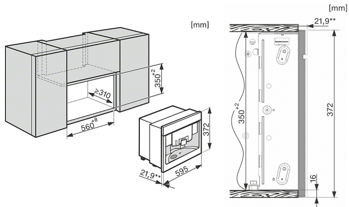
CVA6431ed i överskåp, (skiss) (fotnot)
