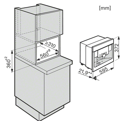
CVA6431ed i utbyggnadsskåp (skiss) (fotnot)
