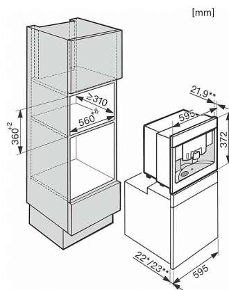
CVA6431ed högskåp och ugn (skiss) (fotnot)
