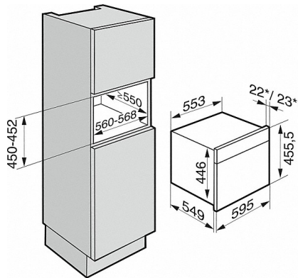
DG 6000 i högskåp (skiss) CH
