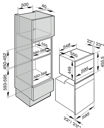
DGC 6500, DGC 6600, DGC 6800, DGC 6805, i högskåp i kombination med ugn, CLST (skiss)
