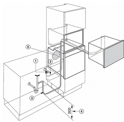
DGC 6805, vattenanslutning (skiss)
