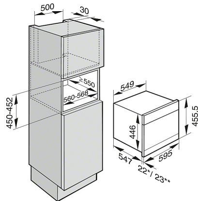
DGC 6300, DGC 6400, i högskåp, CLST (skiss)
