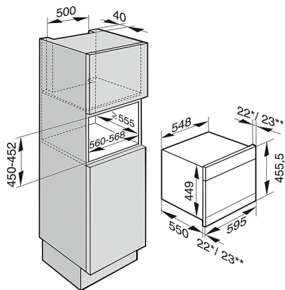
DGC 6500, DGC 6600, DGC 6800, DGC 6805, i högskåp, CLST (skiss)
