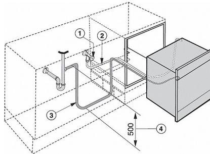
DGC 6000 i underskåp, CLST (skiss)
