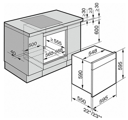
DGC 6000 i underskåp, CLST (skiss)
