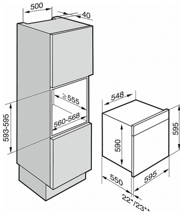
DGC 6000 i högskåp, CLST (skiss)
