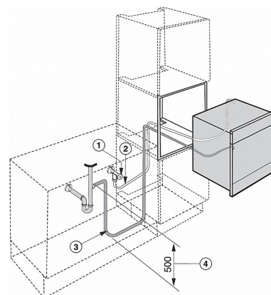
DGC 6000 i högskåp, CLST (skiss)
