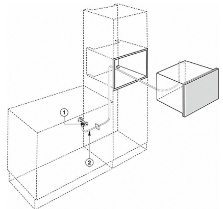
DGM 6000 - vattentillopp (skiss)
