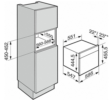
DGM 6000 (skiss)
