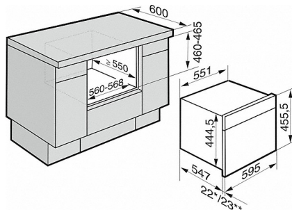
DGM 6000 (skiss)
